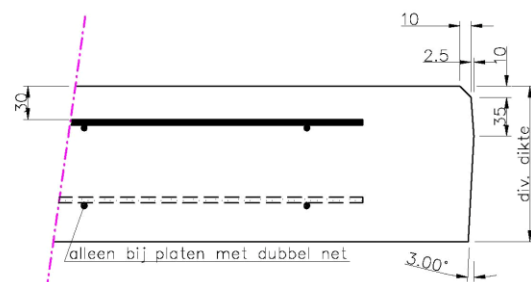
Doorsnede A
