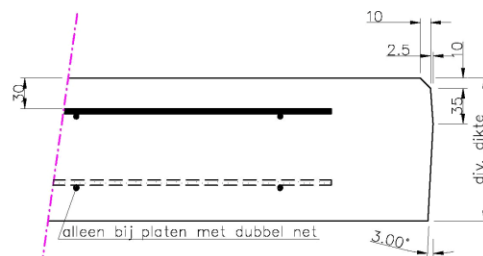
Doorsnede A
