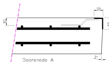
Doorsnede A
