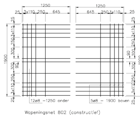
Wapeningsnet 802 (constructief)
