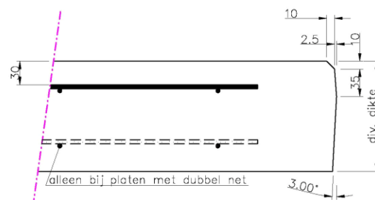
Doorsnede A
