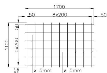
Wapeningsnet 504 (niet constructief)
