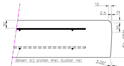
Doorsnede A
