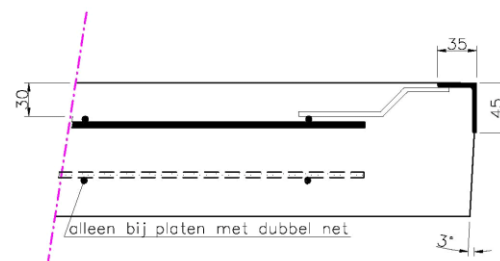
Doorsnede A
