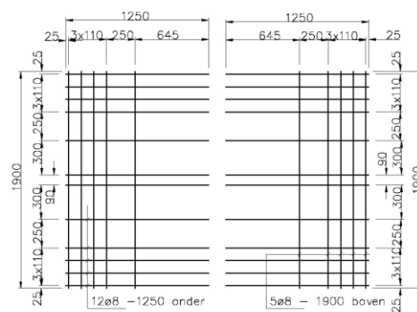
Wapeningsnet 802 (constructief)
